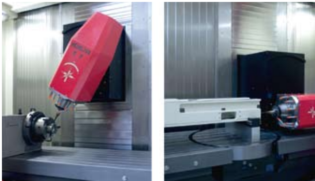
Centre d'usinage combiné à 3 et 5 axes à montants mobiles équipé d'une table rotative et pivotante fixe pour l'usinage simultané sur 5 axes.
